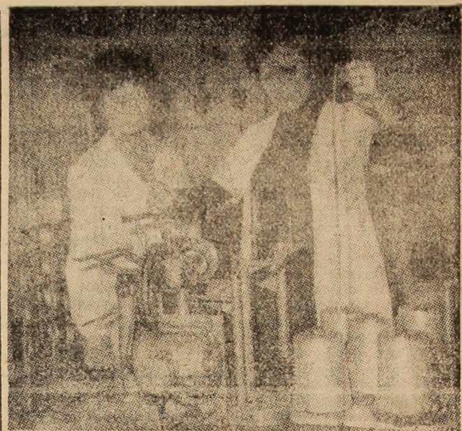
Laboratorul textil de la I.F.A. Viscoza Lupeni, unde Adriana Pușcașu și Iuliana Hiesch determină rezistența mecanică a firului de mătase artificială.
