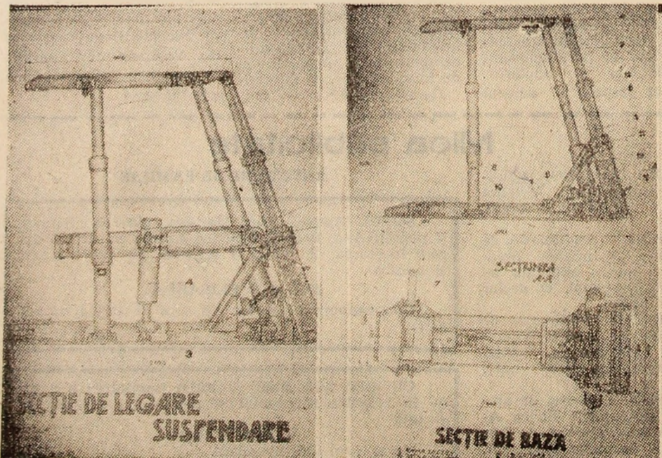
Cadru de susținere al unui complex mecanizat folosit în premieră la I.M. Petrila. Rezultatele obținute confirmă și îndeamnă la generalizarea experienței câștigate.
