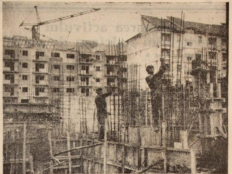
În cartierul Petroșani-Nord, formația de dulgheri condusă de Gheorghe Neagoe pregătește cofrajele pentru turnarea betoanelor în diafragma blocului 81.
