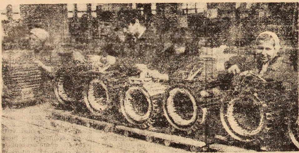
Linia de lucru „în flux continuu” din cadrul secției bobinaj de la I.P.S.R.U.E.E.M., unde se rebobinează motoare electrice de diferite puteri.
