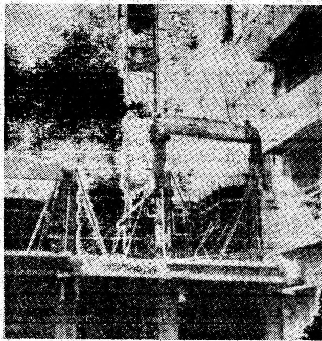
Constructorii șantierului din Vulcan înalță un nou tronson al blocului turn 3B din zona noului centru civic al orașului. Foto: N. ȘTEFAN
