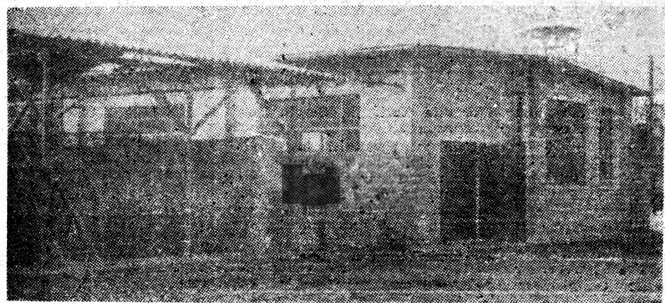
De curînd a fost pusă în funcțiune stația de aeraj de mare capacitate de la puțul auxiliar nr. 2 al L.M. Livezeni. Echipată cu un ventilator avînd o capacitate de 6000 mc aer pe minut, dotată cu dispozitive automate de înregistrare și măsurare a presiunii și debitului, noua și modernă stație contribuie la îmbunătățirea aerajului general al minei.
