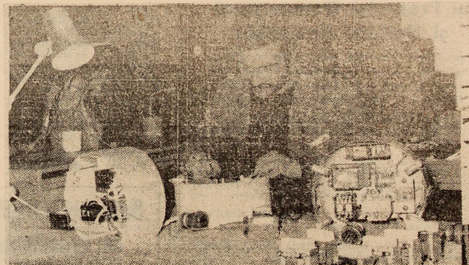
Electronistul Ioan Chirvas din cadrul atelierului de automatizări al IPSRUEEM efectuează testări la un nou produs asimilat „Adaptor de comandă pentru telegrizometrie — ACT”. Foto: Ion BĂLOI
