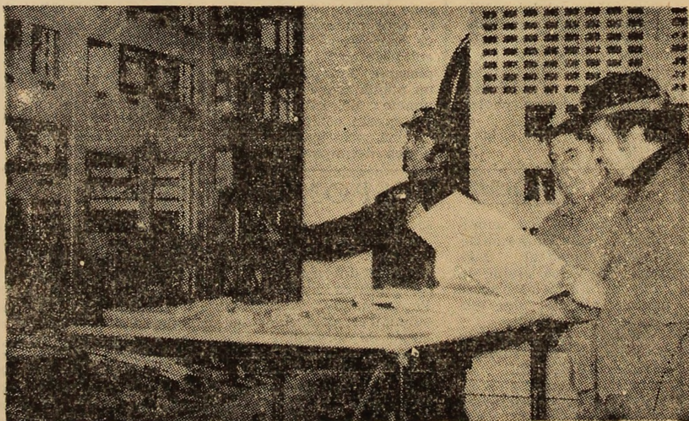
Camera de comandă tehnică a cazanului nr. 1 U.E. Paroșeni. Maistrul Gheorghe Mirea și electricienii Ion Militaru și Radu Udrouiu (Energomontaj București) lucrează la modernizarea instalației de automatizare.
