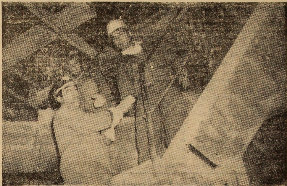
Antrepriza în zidiri refractare — București, brigada Cluj-Napoca, condusă de ing. Adrian Balint și ing. Florea Barbu, execută lucrări de calitate la cazanul nr. 1 de la Uzina electrică din Paroșeni. Foto: Al. TĂTAR
