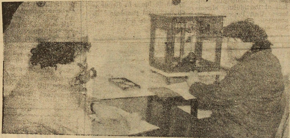
Maria Sicoe și Ioana Eleonora — laborante C.T.C., lucrînd la determinarea conținutului de cenușă la probele cărbunelui brut extras la I.M. Lupeni.
