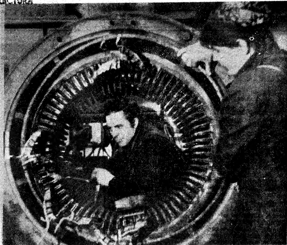
La IPSRUEEM Petroșani, creșteri substanțiale au cunoscut, în acești ani, gradul de înnoire tehnică și nivelul de pregătire profesională a personalului muncitor. În imagine, sub coordonarea maestrului Ioan Neuchoff se execută lucrări de bobinare pentru motoare de mare putere energetică. Foto: I. LICIU
