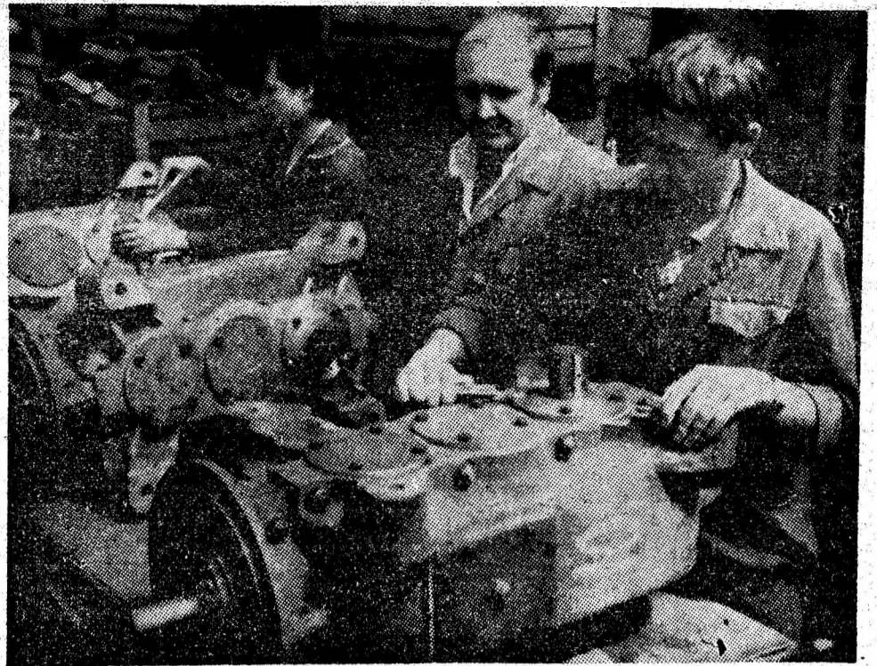
Secția montaj a IUMP. Se lucrează la un nou lot de reductoare pentru transportoarele miniere. Foto: O. GEORGESCU
