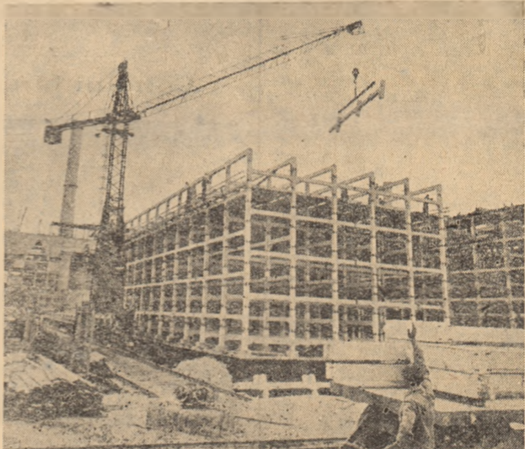
ÎN FOTO: Scheletul din piese prefabricate al ventilatorului de răcire a termocentralei care se construiește la Lübbenau.
