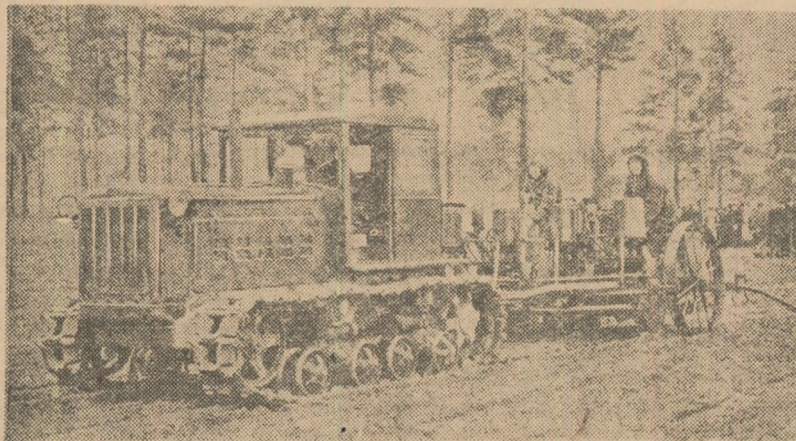
Mașina „S.K.G.-4” pentru plantarea cartofilor prin metoda în cuiburi pătrate. În acelaș timp ea introduce în cuiburi îngrășăminte minerale.
