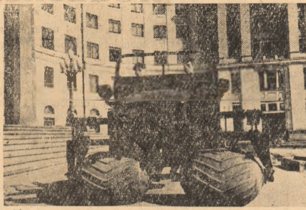
În U.R.S.S. s-a realizat o instalație autopropulsată experimentală care servește la încercarea noilor anvelope fără cameră cu presiune foarte joasă. Aceste anvelope de tip nou vor fi folosite la vehiculele pentru orice teren. Automobilele înzestrate cu aceste anvelope nu se tem de drumurile impracticabile, ele putînd circula pe nisip și zăpadă. În foto: Vedere de ansamblu a mașinii experimentale.
