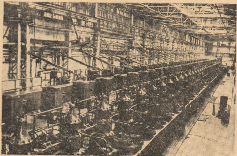
La Fabrica de sticlă „F.E. Dzerjinski” din Gus-Hristalnoi U.R.S.S. se procedează la reorganizarea transportorului de șlefuire și lustruire a sticlei, spre a asigura o funcțiune continuă. În foto: În secția fabricii — transportorul principal de șlefuire și lustruire a sticlei.
