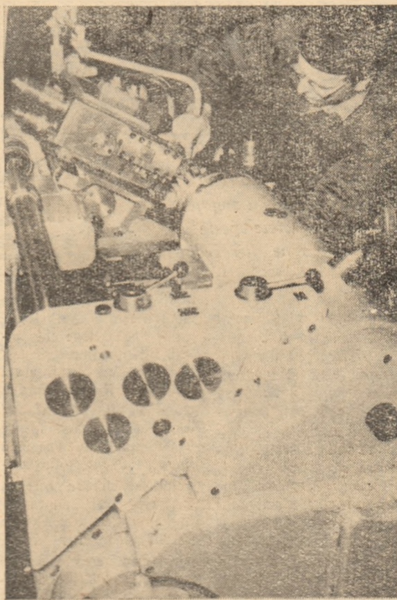
Mașina-unealtă „I2S 200x6“ de tăiere automată a cablurilor produse în R. S. Cehoslovacă.
