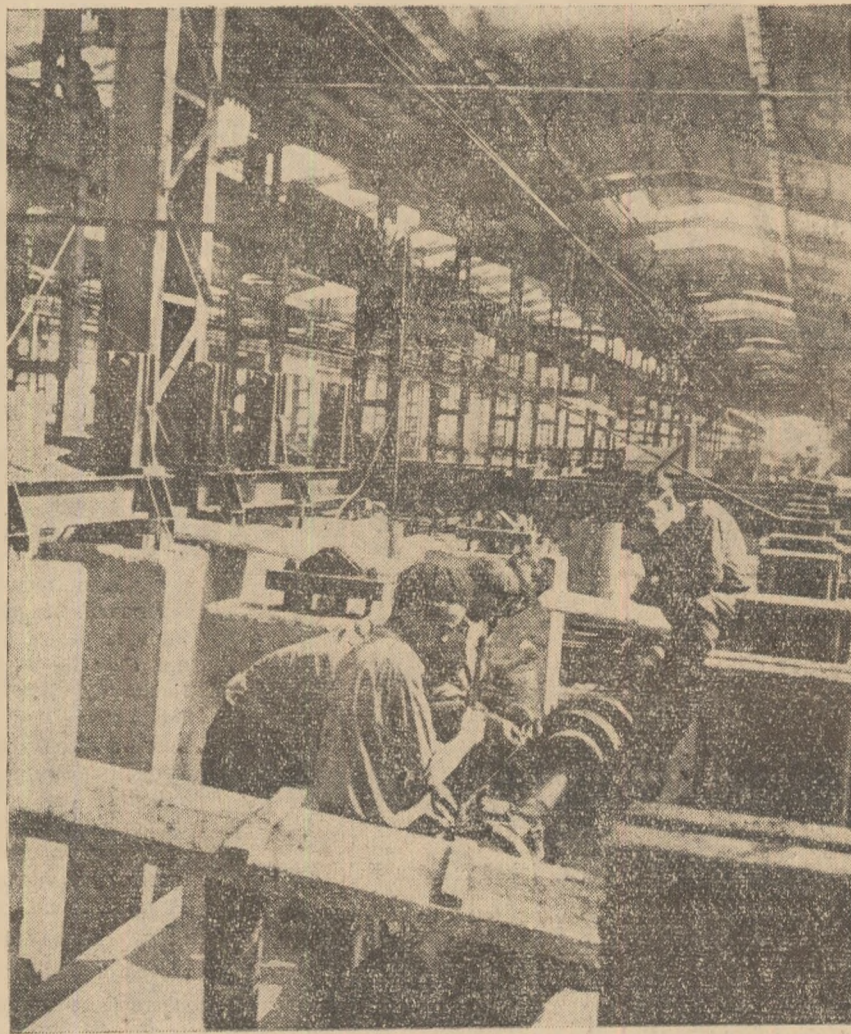
Lucrările efectuate de constructorii I.C.S.H.-ului la laminorul de profile mici și mijlocii sînt destul de avansate. De curînd a început montarea agregatelor la linia de sîrmă care va fi dată în folosință nu peste multă vreme.
