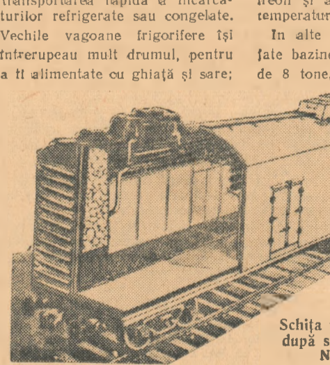
Schița unui vagon frigorifer după sistemul inginerului N. A. Kleimenov
