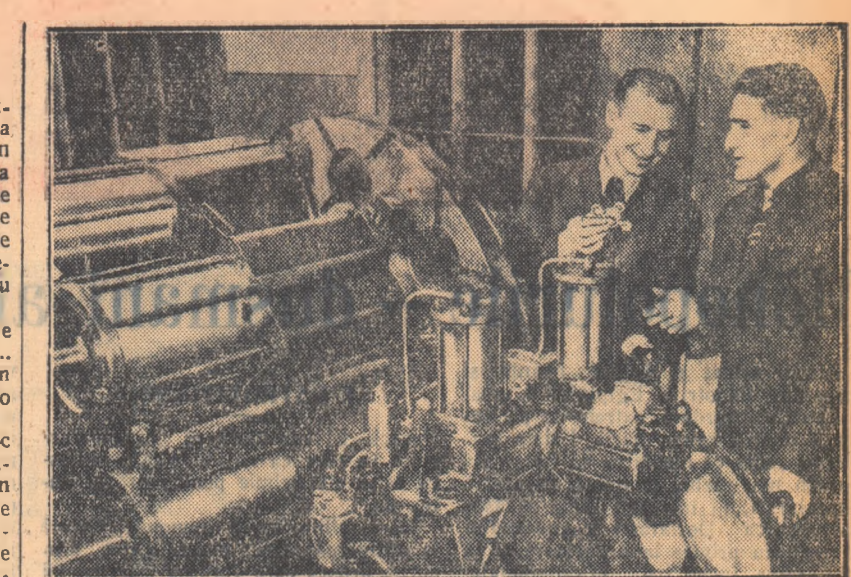
La Institutul de cercetări științifice pentru tehnologia construcției de mașini din Moscova s-a construit un nou automat pentru turnarea precisă a pieselor. Într-o oră se pot turna 800-1.500 de piese, avînd fiecare o greutate de 30-200 de grame. Iată-i pe Ing. V. Zimin (stînga) și Ing. V. Tarasov verificînd funcționarea automatului. Fețele lor mulțumite dovedesc că așteptările nu le-au fost înșelate.
