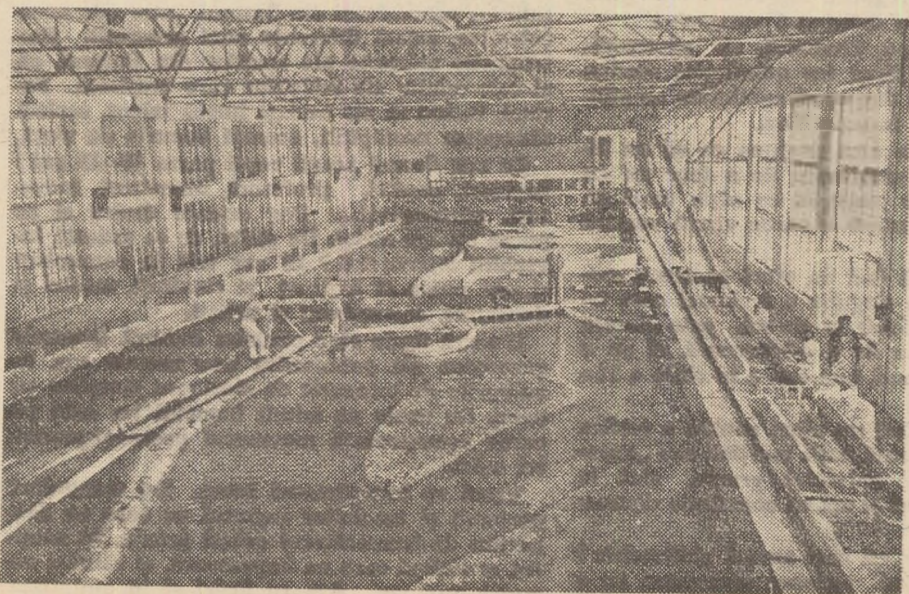
Un riu în miniatură într-un laborator al Institutului de cercetări științifice pentru hidrotehnică și îmbunătățiri funciare din R.S.S. Gruzîni
