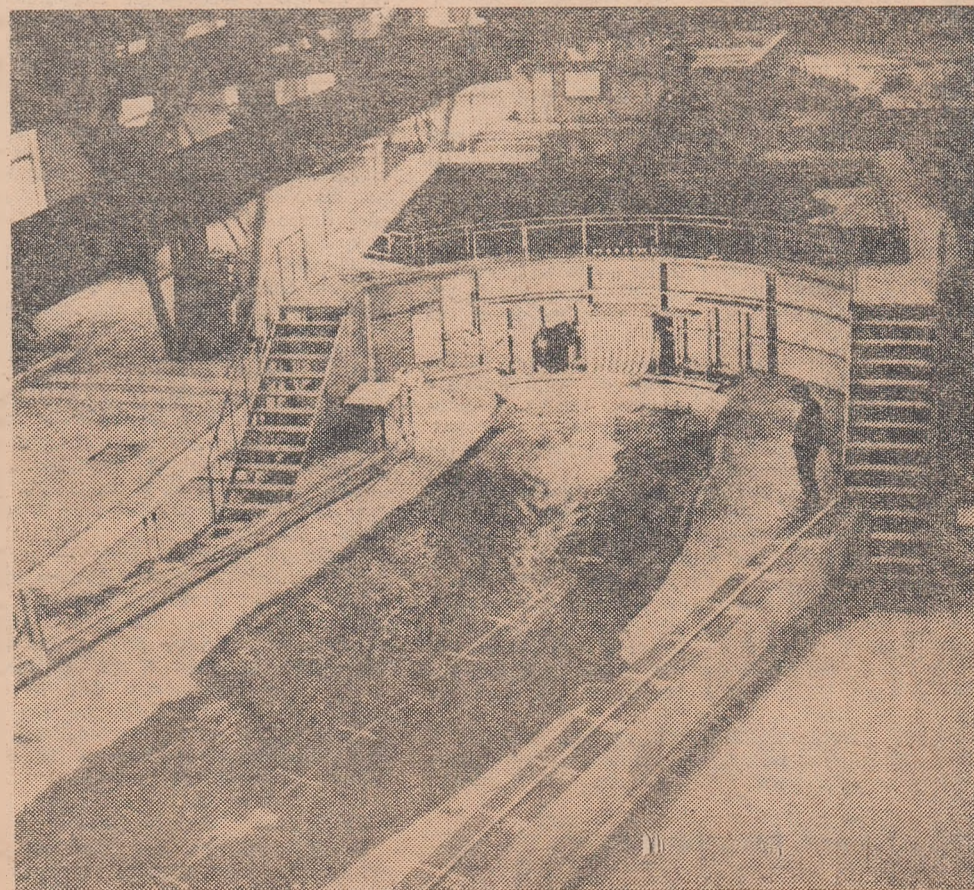
Impresionanta machetă a hidrocentralei Saian — Șusenskoie
