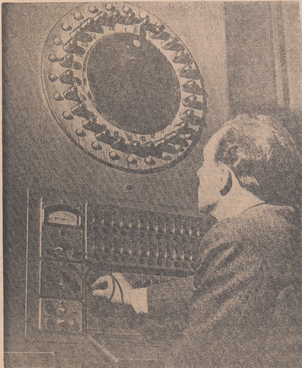
Instalație pentru măsurarea la distanță a radiației gama în centralele atomoelectrice
