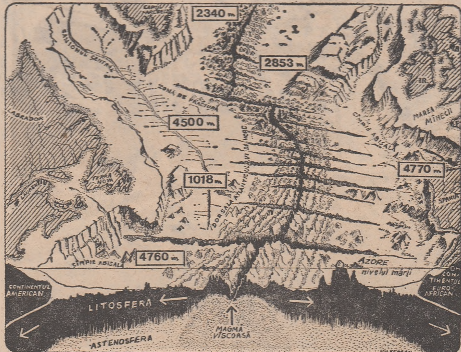
Dorsala medio-atlantică, așa cum se prezintă ea în partea de nord a oceanului. Între cele două „buzi” muntoase, riftul în care urcă magma din adîncul Terrei
