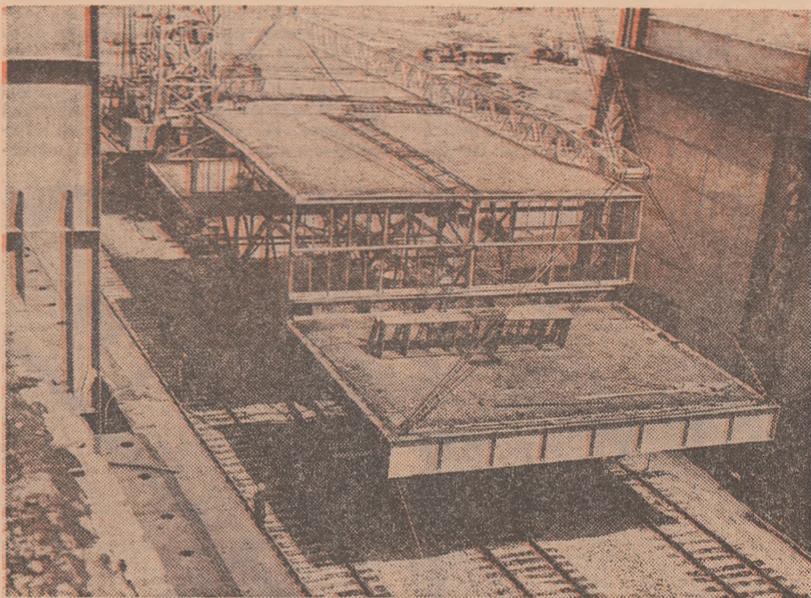
La Ceboksari, capitala R.S.A. Ciuvașe, se construiește o uzină de tractoare industriale de 220, 330 și 500 CP. La construcția noii întreprinderi se utilizează panouri de 360 de metri pătrați, asamblate pe conveier. În felul acesta productivitatea muncii constructorilor a sporit cu 40 la sută. În fotografie: Asamblarea unui panou pentru planșeu
