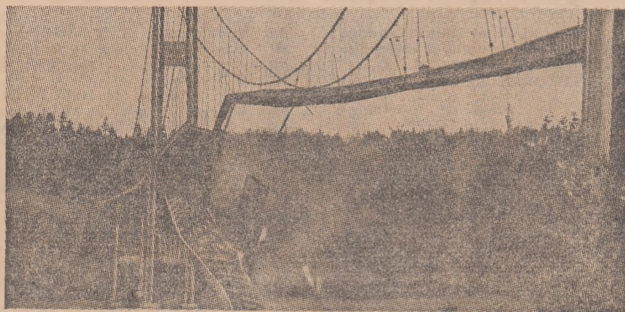
Podul din Tacoma, statul Washington (S.U.A.), a fost construit fără probe prealabile într-un tunel aerodinamic. La 11 septembrie 1940, o puternică rafală de vînt a dat naștere la presiuni și fenomene de rezonanță, care l-au făcut să se prăbușească.
