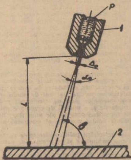
Fig. 2 1. diuză 2. semifabricat
